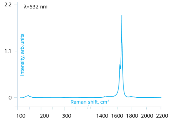
TUBALL™ ラマンスペクトル (標準CNT)
