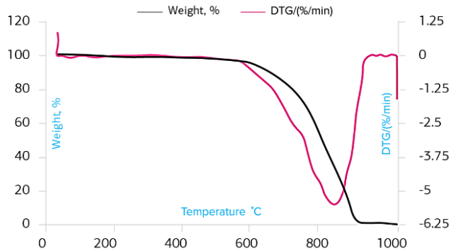
TUBALL™ TGA曲線 (精製CNT)
